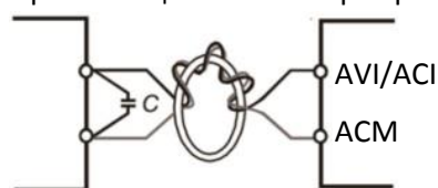
Ферритовое кольцо
